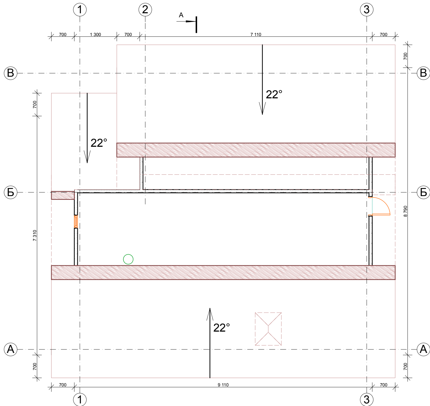
План кровли
